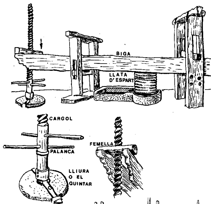
Figures 30 i 31 Premsa de biga o de «lliures» Museu del vi de Vilafranca del Penedès (Fig. 30) Premsa medieval derivada del tòrcul romà. Manuscrit d'Albucassis, traducció del segle XIV. Segons DUBY et alii, Histoire de la France . Mateix tipus de premsa a la Touraine del segle XVIII (Fig. 31) Aquestes premses són imitades del tòrcul romà. Eren utilitzades a Catalunya a les planes baixes, fins al segle XIX.
