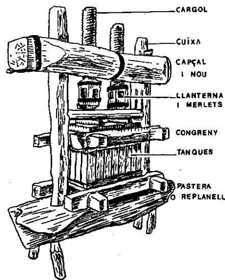
Figura 33 Premsa de doble cargol descendent. Premsa presentada al Museu del vi de Vilafran- ca del Penedès. En aquest exemplar del se- gle XVIII, es noterà un sòcol de fusta sobrealçat molt di- ferent del precedent sòcol de pedra amb tasconera lateral.
