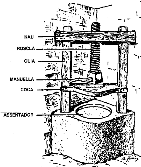
Figura 37 Premsa de sagristia. Eivissa segons ALCOVER I MOLL. Localitzades en un racó del celler, aquestes petites premses servien per a espremer el darrer suc d'una collita ja trepitjada dins un cup de fusta.
