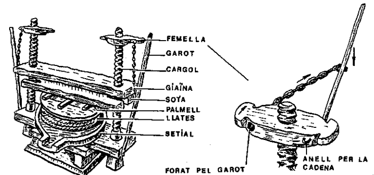
Figura 34 Premsa de garrot (segons F. POIROT, 1973) Premsa emprada al Rosselló, probablement a partir de la Renaixença. Un enginyós sistema de palanca permetia de fer girar la femella entorn dels dos cargols laterals. El sòcol és de fusta.
