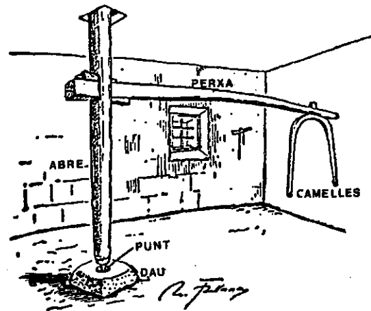
Figura 42 Molí de sang mallorquí (segons ALCOVER I MOLL). Aquesta presentació d'una enginyeria de molí demostra que el sòcol de pedra no és mantingut al terra per cap sistema de fixació. La seva forma quadrangular li permet de mantenir-se immòbil.
