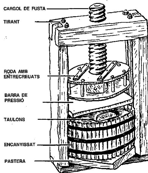
Figura 38 Premsa de cargol descendent. Exemplar rossellonès de final del segle XIX (segons POIROT, 1973). Aquesta premsa, reforçada per una xarxa de filferro, marca l'última evolució de les premses de cargol descendent.
