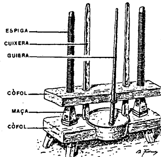
Figura 39 Premsa de dos cargols laterals. Mallorca segons ALCOVER I MOLL. Aquesta premsa, de la qual només s'ha conservat l'enginyeria de fusta i de ferro, mostra una variació original i tardana de la premsa de dos cargols laterals. Són mòbils com per les premses de cargol descendent.
