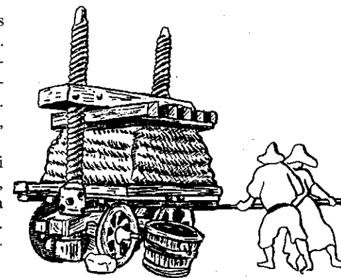
Figura 40 Premsa ambulante de dos cargols laterals mòbils. Utilitzada al Llenguadoc al segle XIX (segons un dibuix de C.L. HORA SICCAMÀ, 1848). La collita era premuda i donava un primer suc, després era trepitjada dins pasteres de fusta. En fi la brisa era acordonada i premsada.
