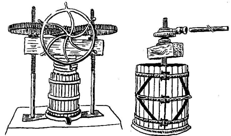
Figures 35 i 36 Premsa de volant i premsa de mà actual. (Museu del vi de Vilafranca del Penedès - La Bisbal). Aquestes premses mecàniques amb enginyeria de ferro evidencien l'evolució del sistema de dos cargols i femella descendents. Els sòcols poden ésser de pedra, els més senzills, o de ferro com aquí.
