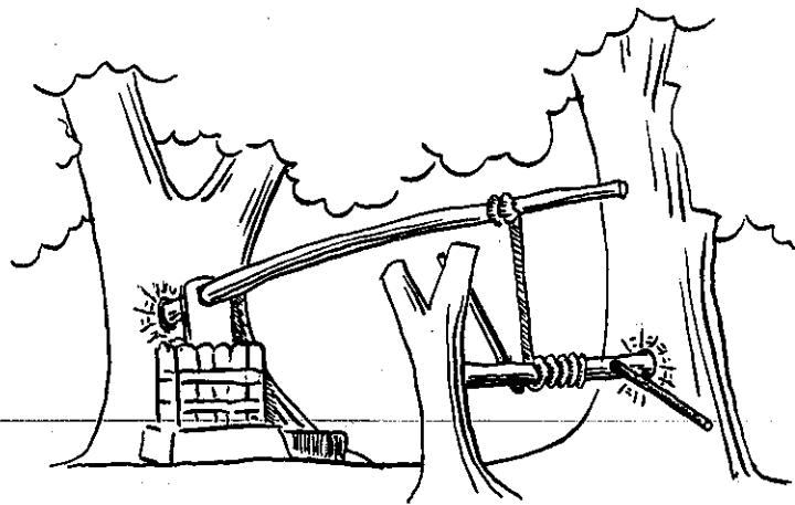
Figura 41 Premsa de vi amb palanca i torniquet. Aquest exemplar de premsa de l'Empordà (CARRERAS I CANDI, 1930), és molt original, puix que utilitza la mateixa tècnica que la de certes premses de formatges. El sistema de «cabrestant» substitueix aquí el contrapès de pedra.
